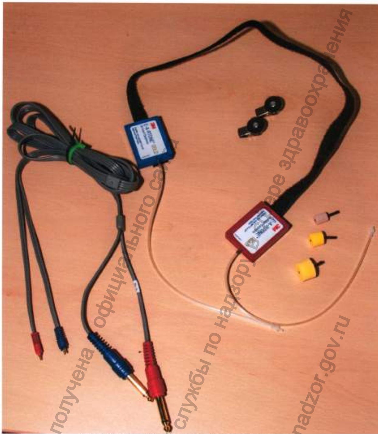
Телефоны аудиометрические внутришние
